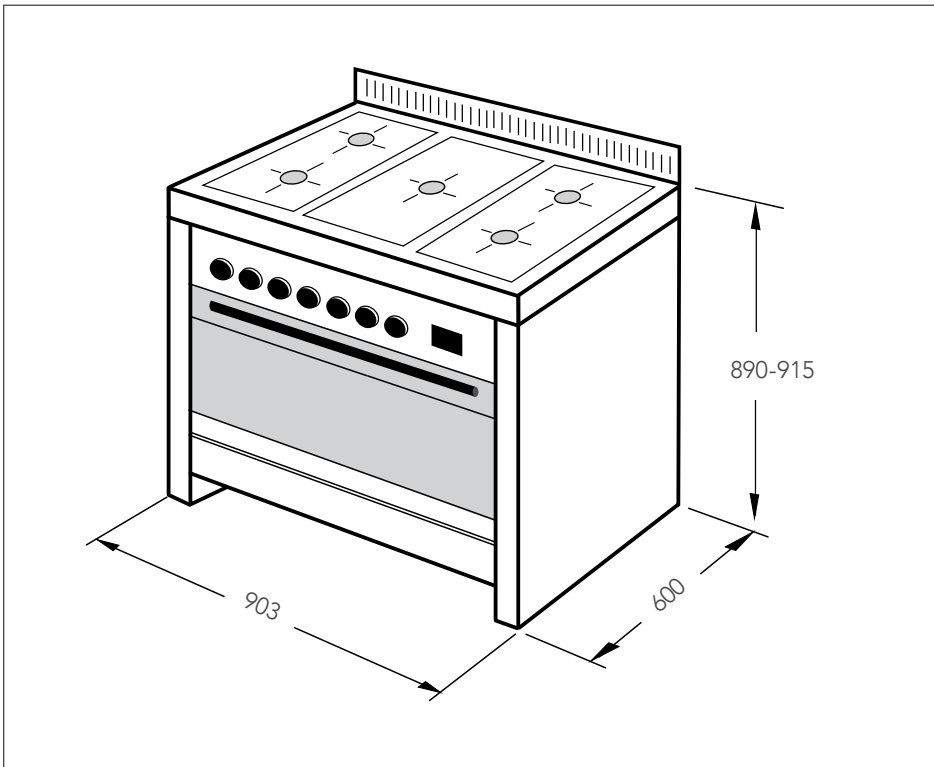
SCU900 UPRIGHT COOKER // 90cm
